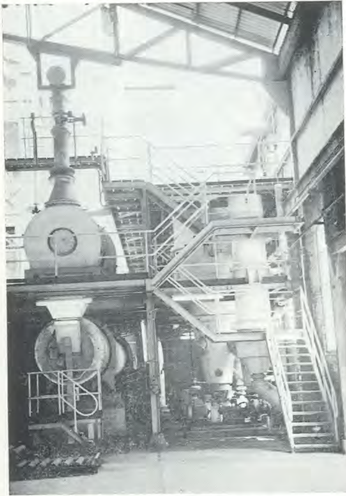
En la nueva unidad de producción de laminitas esta foto recoge lo que pudiera decirse zona de solidificación. En ella aparecen el secador y el refrigerante de laminitas y al fondo, a la derecha, tras la escalera, el evaporador.
