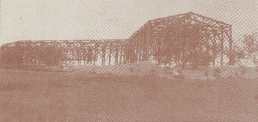
Esta es la estructura metálica de la estación de ángulo que se está montando en La Gándara.
