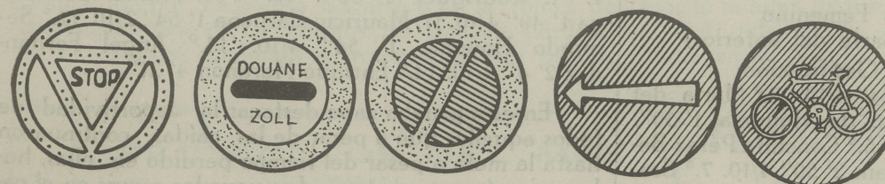
Parada en el cruce (triángulo rojo inscripto en círculo también rojo) Parada (por aduana, arbitrio, etc.) Parada o espera limitada (disco azul, orla roja y franja diagonal roja) Dirección obligatoria (fondo azul, símbolo blanco) Pista obligatoria para ciclista (fondo azul, símbolo blanco)
